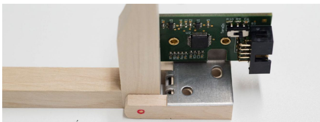
Espressivo-Einzelsensor mit Montagewinkel, Magnet, Trakturwinkel
