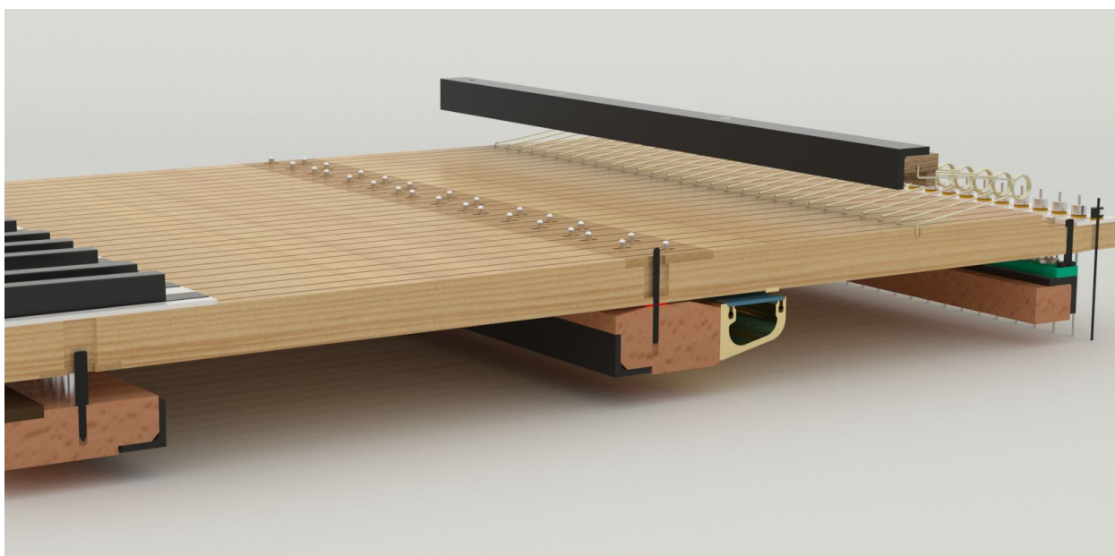
Zweiarmige Klaviatur mit Ruheleiste und invertiert montierter Espressivo-Sensorleiste am Waagbalken.
