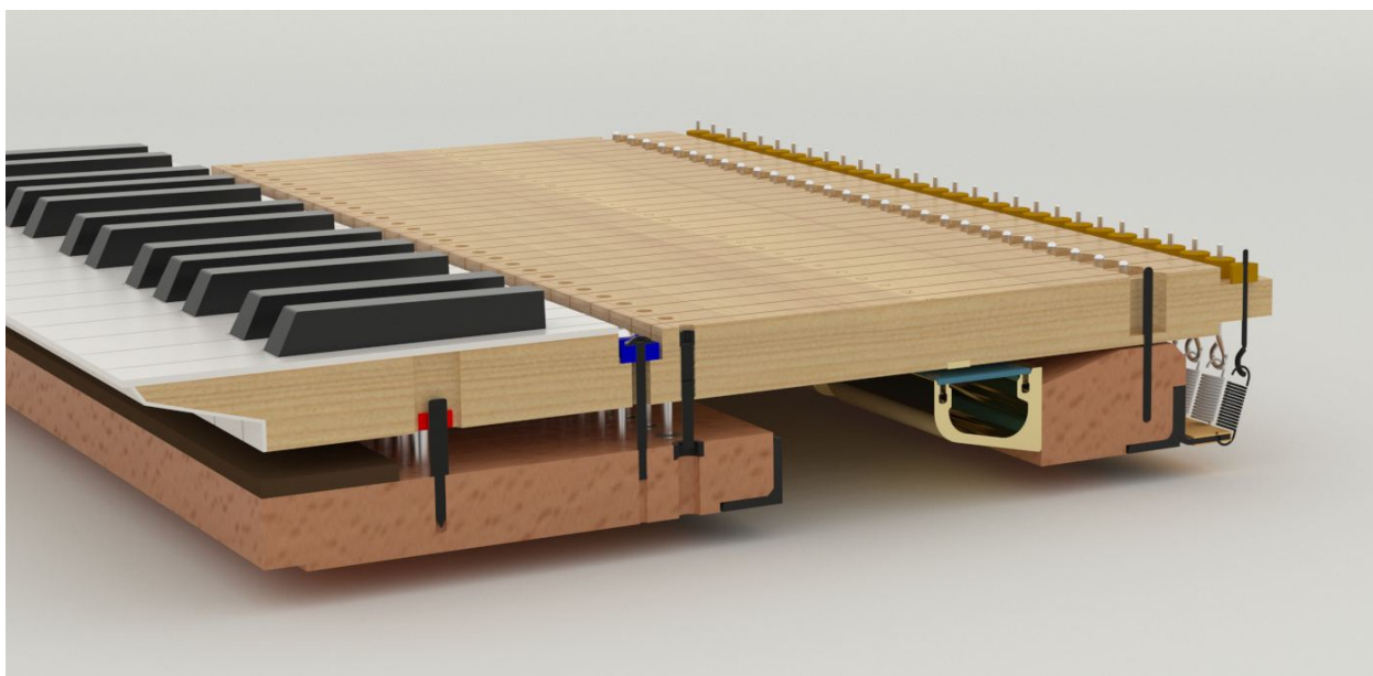
Einarmige Klaviatur mit Druckpunktsimulation und montierter Espressivo-Sensorleiste an der Vorderseite des Waagbalkens.
