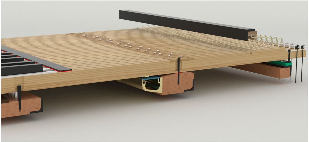
Zweiarmige Klaviatur mit Ruheleiste und montierter Espresso-Sensorleiste an der Vorderseite des Waagbalken.
