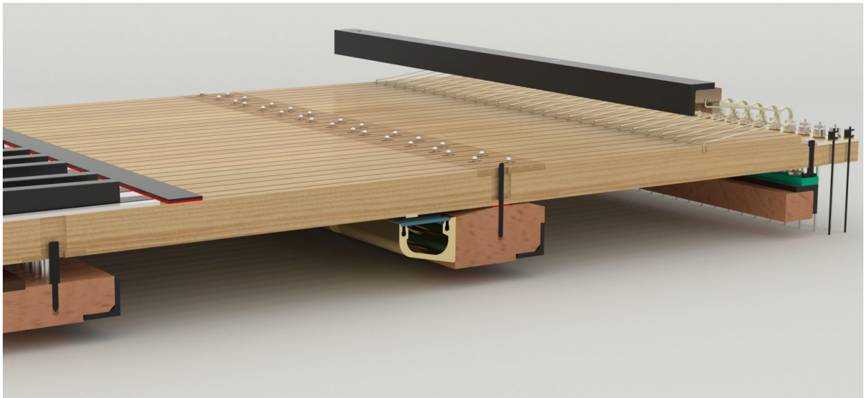
Zweiarmige Klaviatur mit Ruheleiste und montierter Espresso-Sensorleiste an der Vorderseite des Waagbalken.
